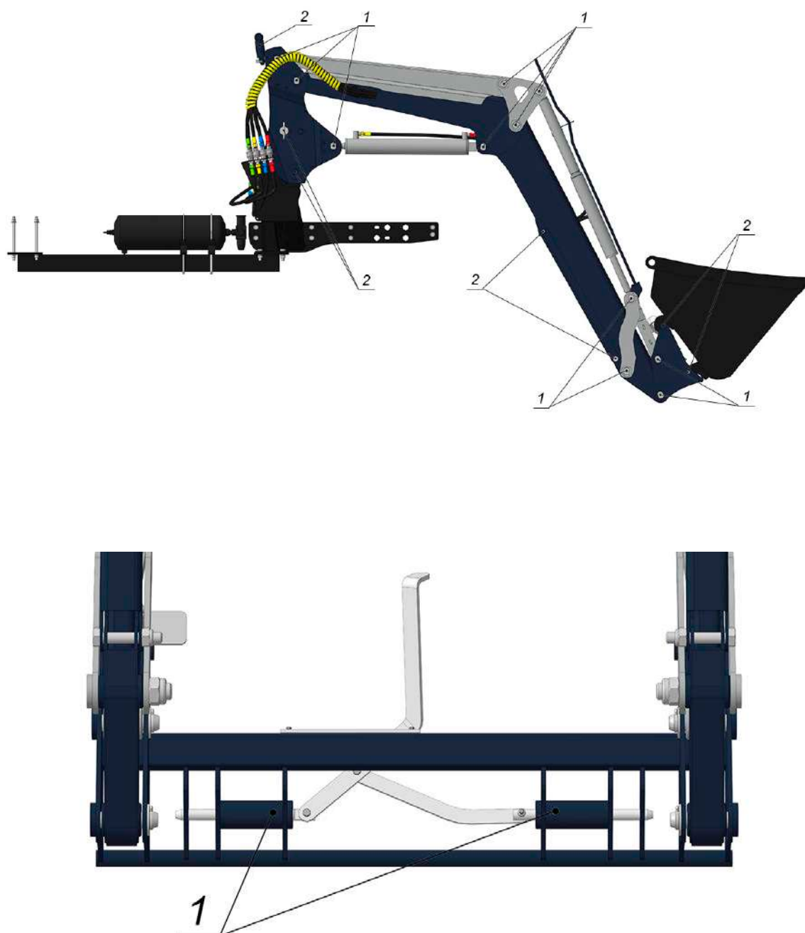
Рис. 3.1 – Схема смазки
