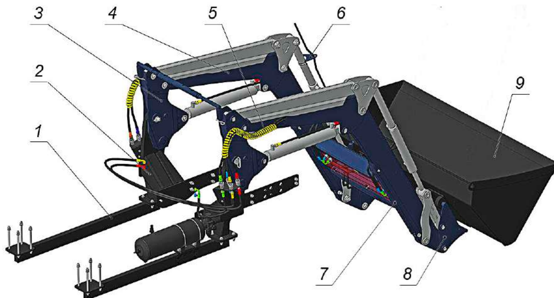
Рис. 1.9 – Общий вид
