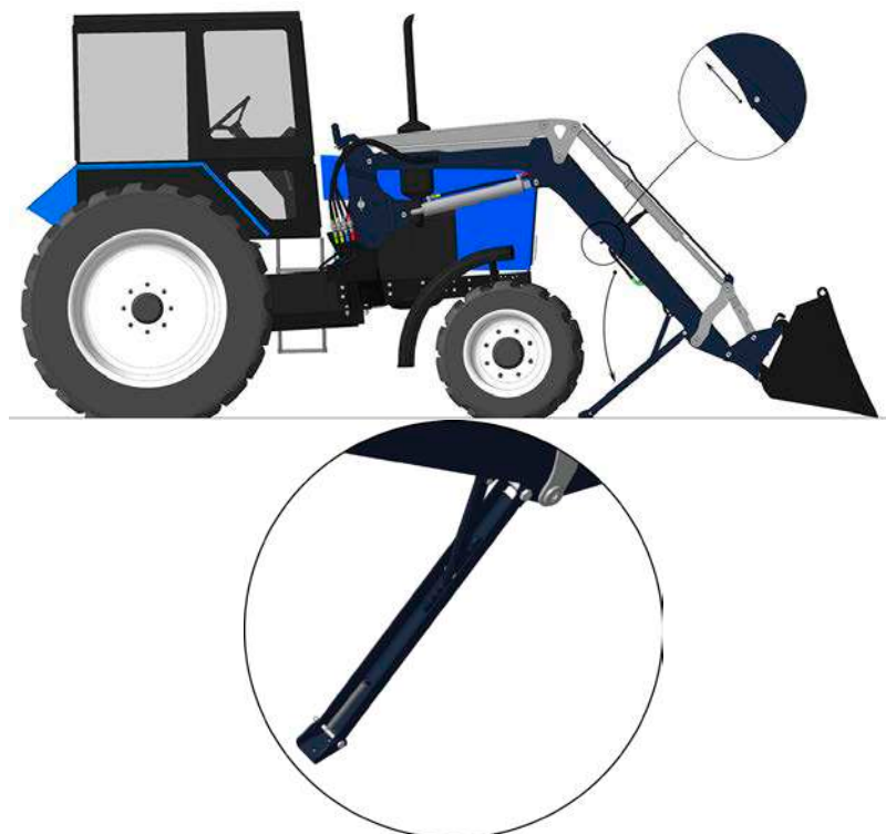
Рис. 2.3 – Опускание упоров на землю
