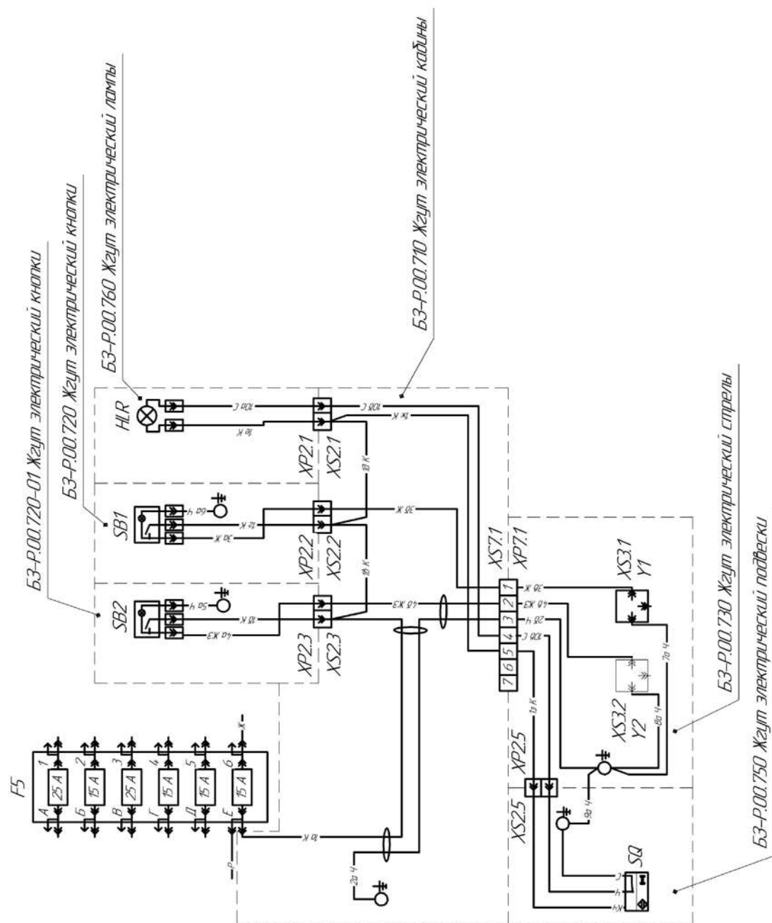
Рис. 6.2 – Комплектация с двумя диверторами без джойстика
